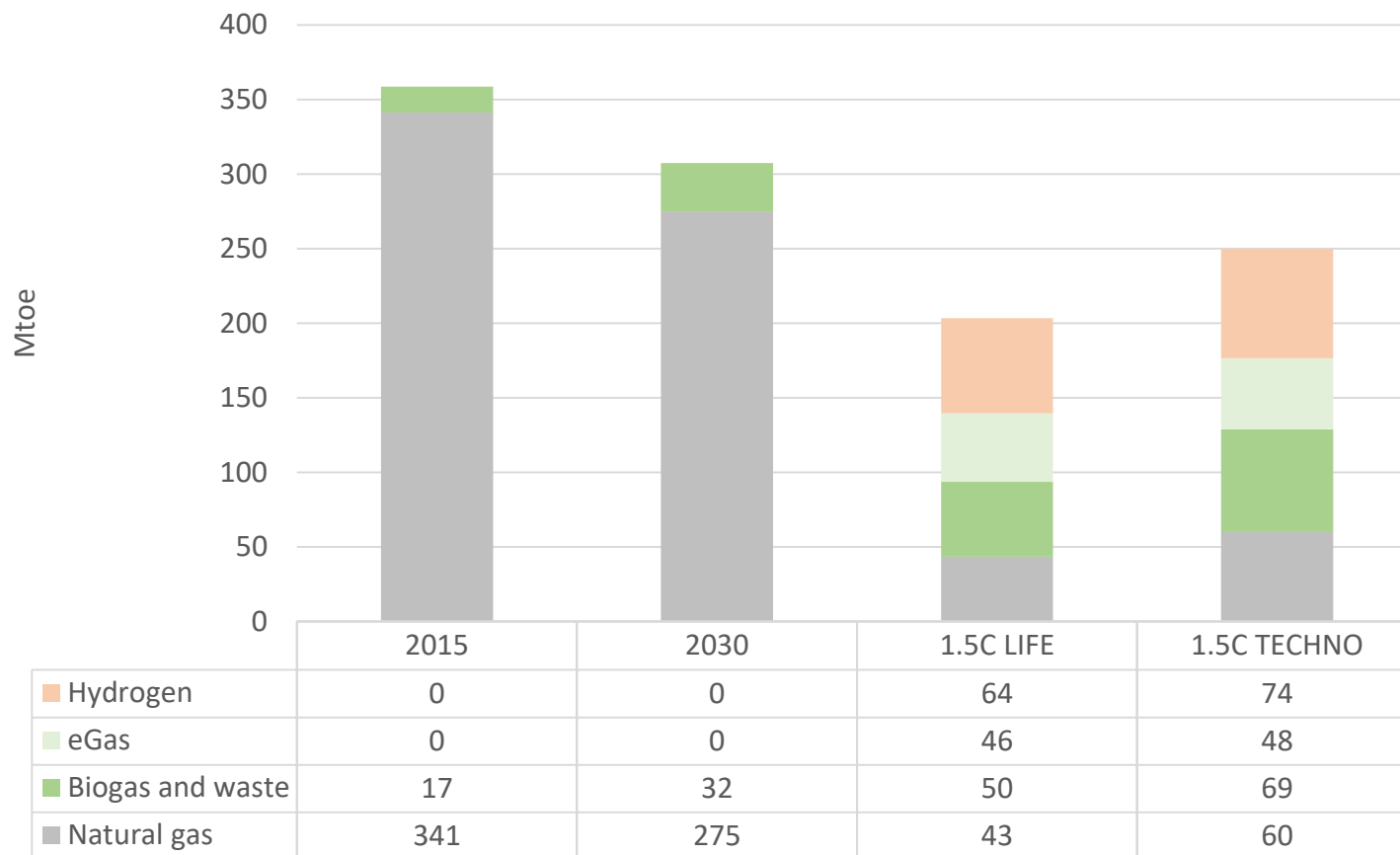
Consommation d'énergie final par vecteur gaz dans les trajectoires de décarbonation compatibles avec les objectifs de l'accord de Paris.
